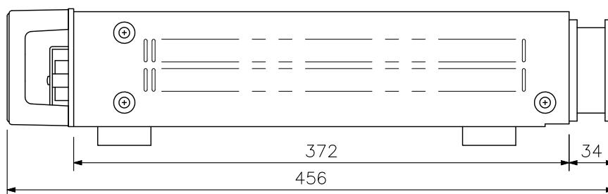
側面図
