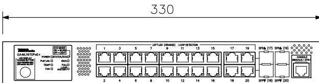
正面図
