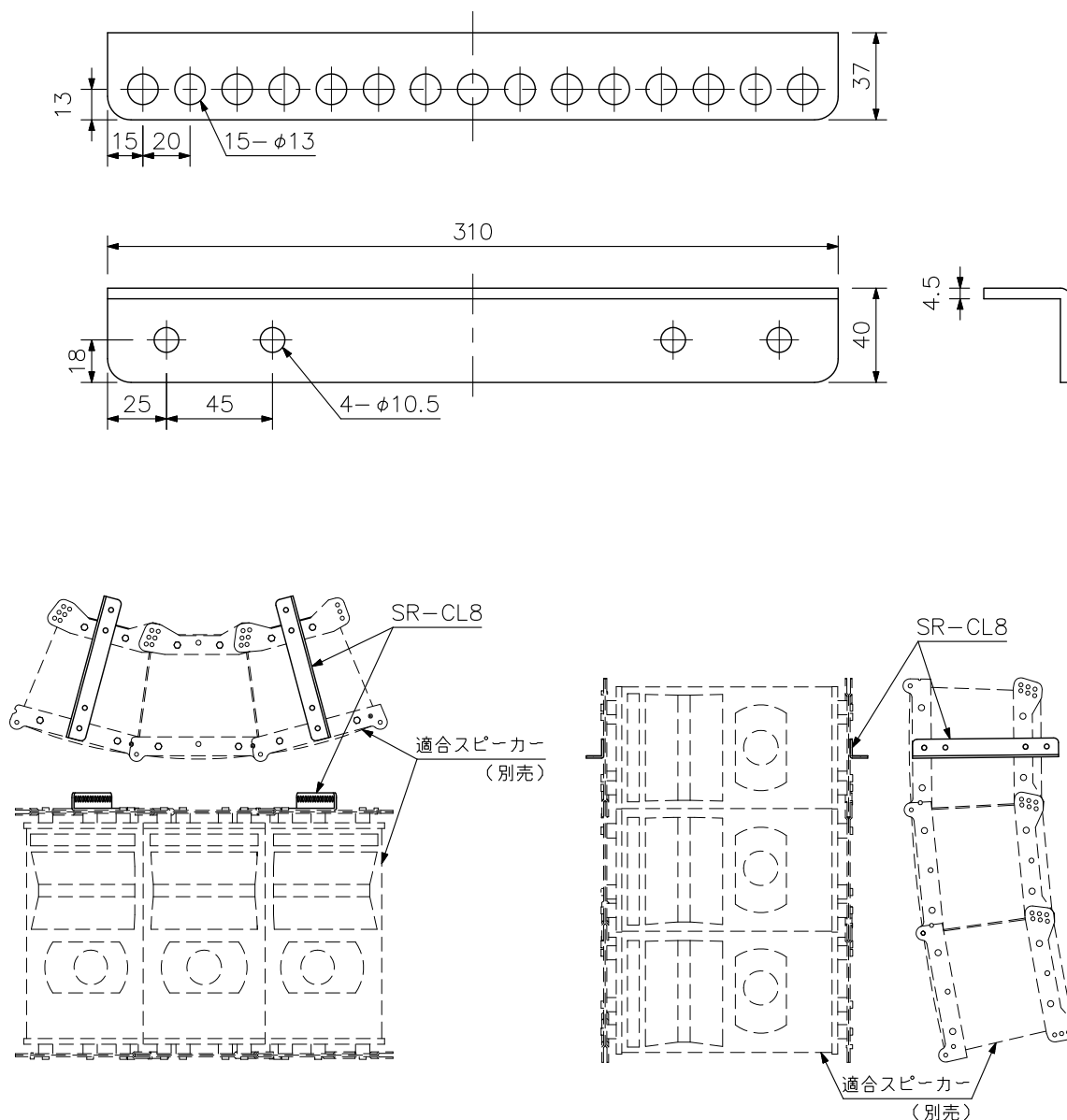
フライング使用例 (縮尺: 1/15)
