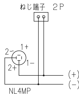
結線図
