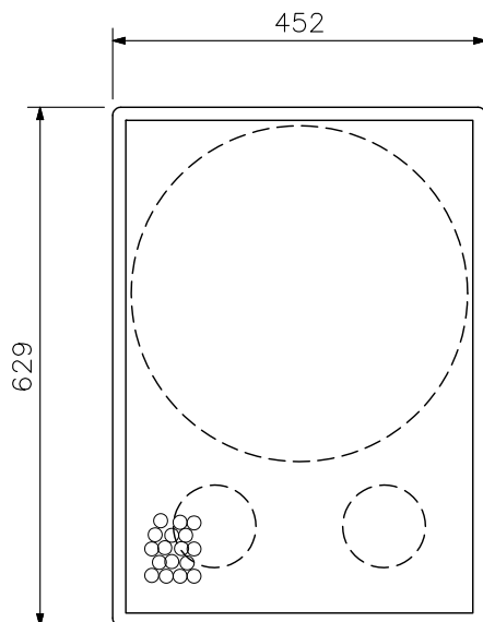
正面図
