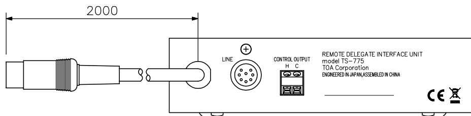
背面図
