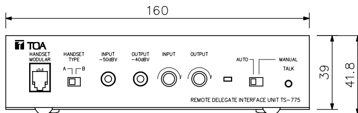
正面図
