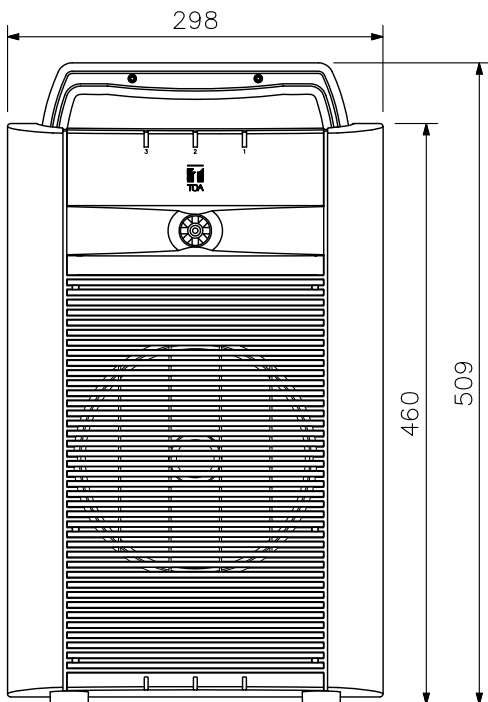
正面図
