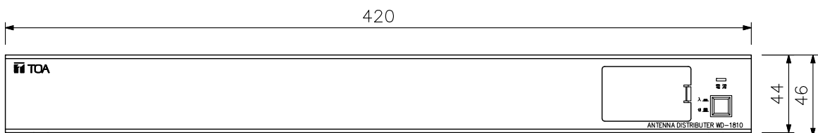
正面図
