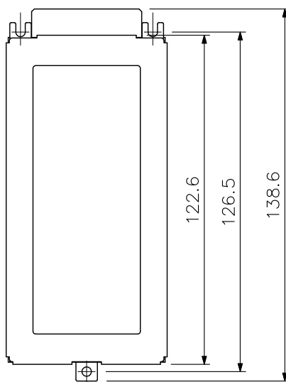
上面図
