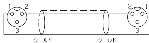
回路図
