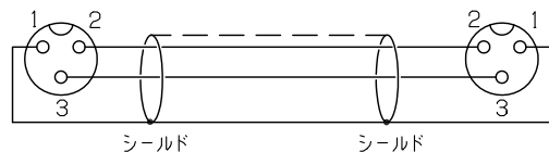
回路図
