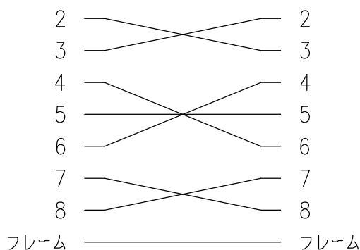
結線図
