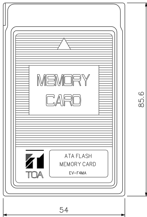
正面図
