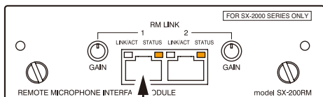
SX-200RM
